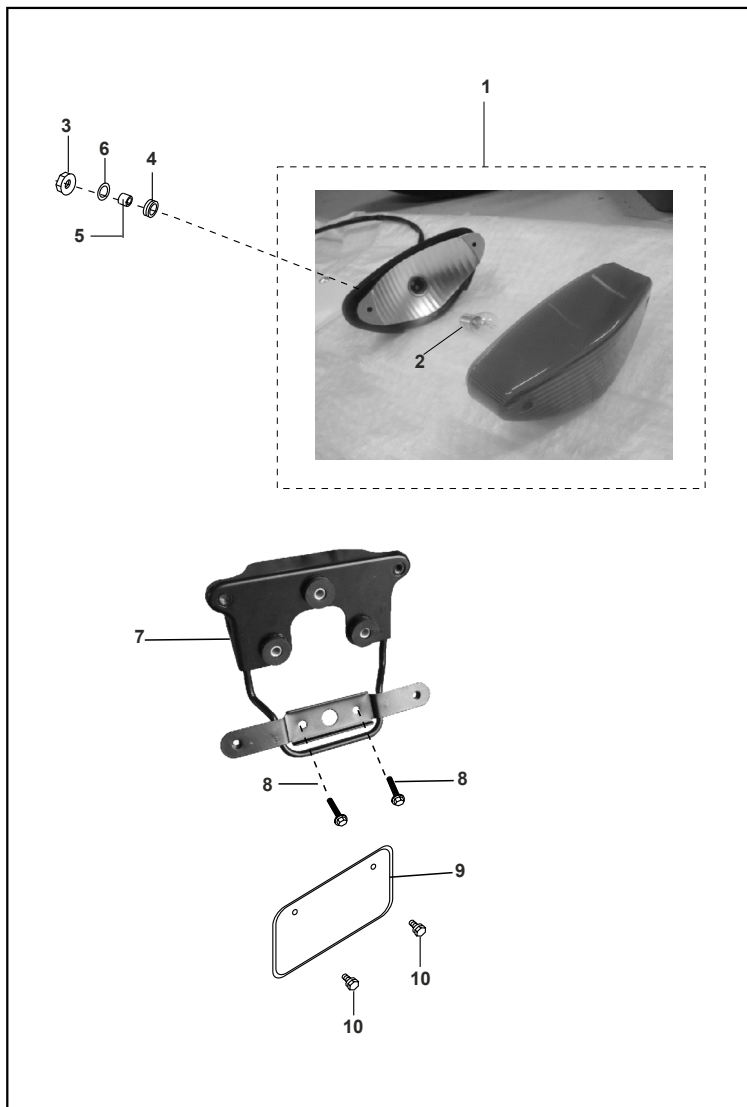
FIGURA N° 40 : STOP
