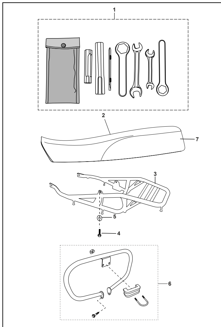
FIGURA N° 42 : HERRAMIENTAS / ACCESORIOS
