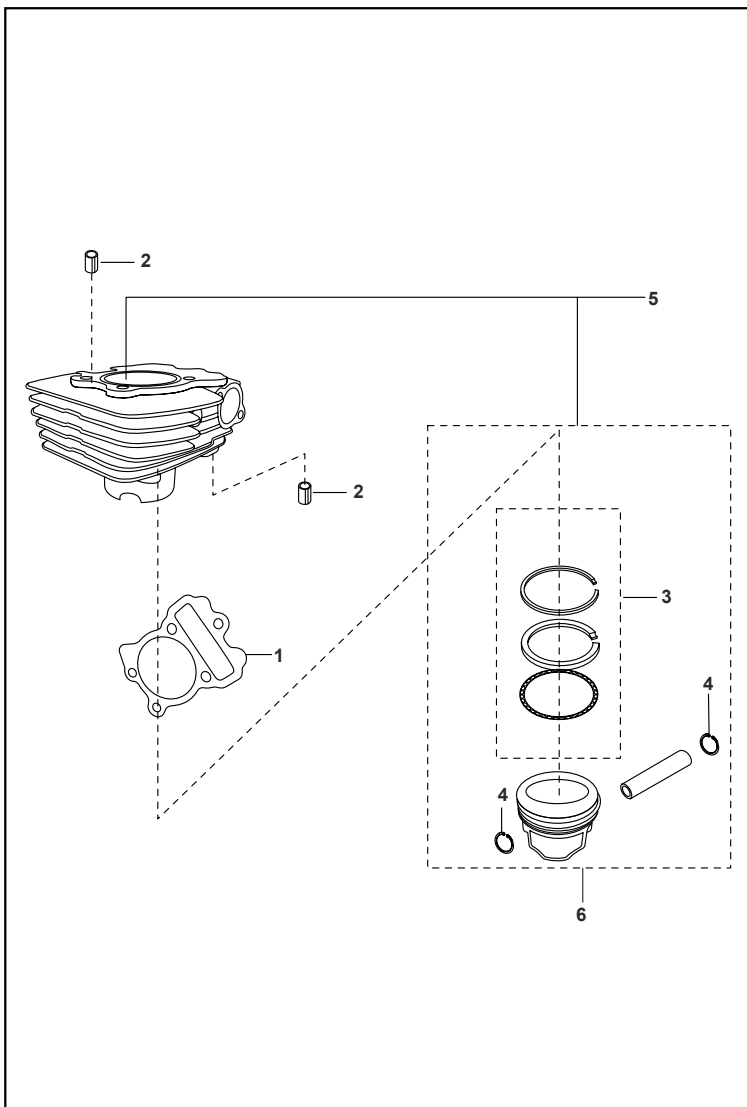
FIGURA N° 5 : CILINDRO / PISTÓN
