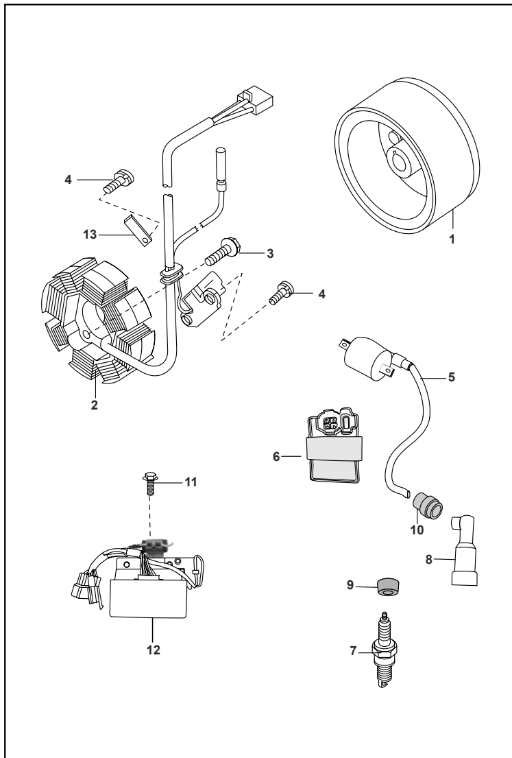
FIGURA Nº 21 : MAGNETO / C.D.I. / PLATO DE BOBINAS
