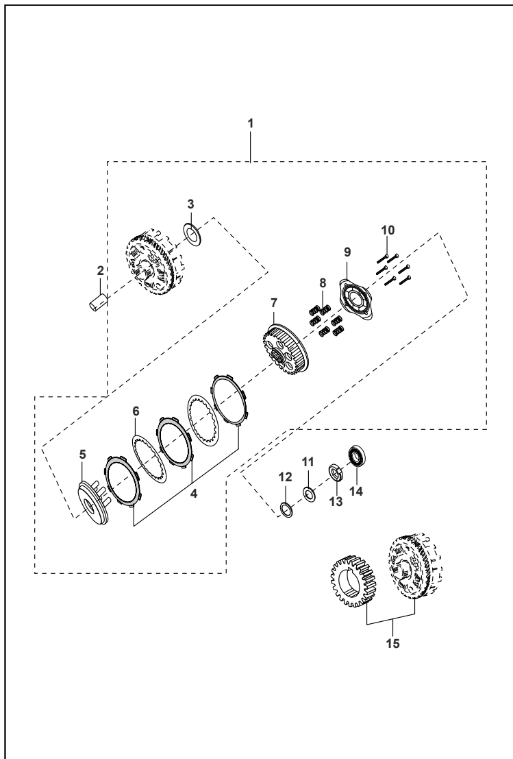
FIGURA N° 14 : CLUTCH
