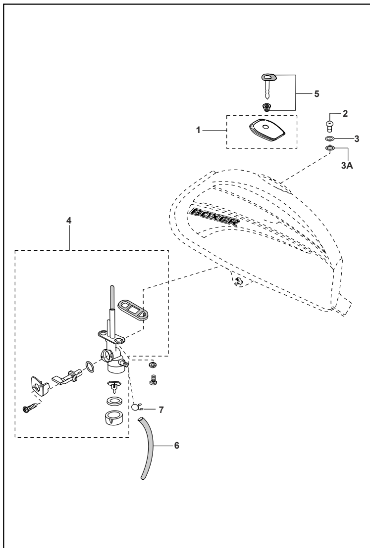
FIGURA N° 34 : GRIFO DE GASOLINA
