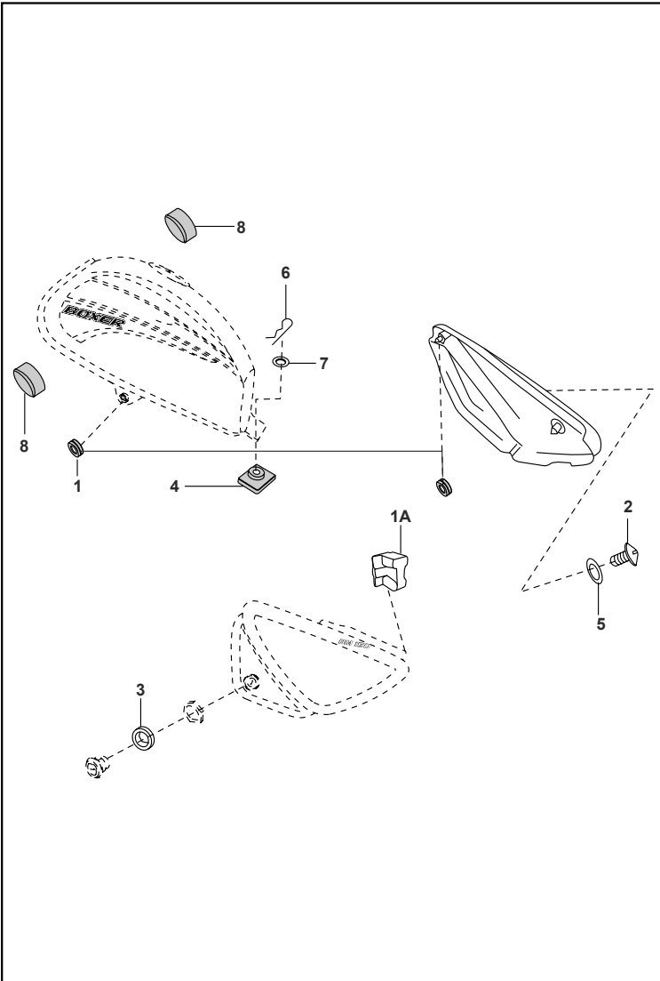
FIGURA N° 33 : ANTIVIBRANTES TANQUE Y TAPAS LATERALES
