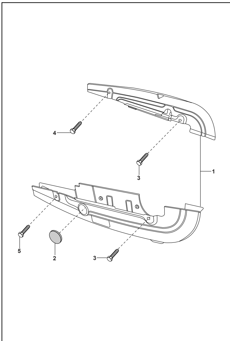
FIGURA N° 35 : GUARDACADENA
