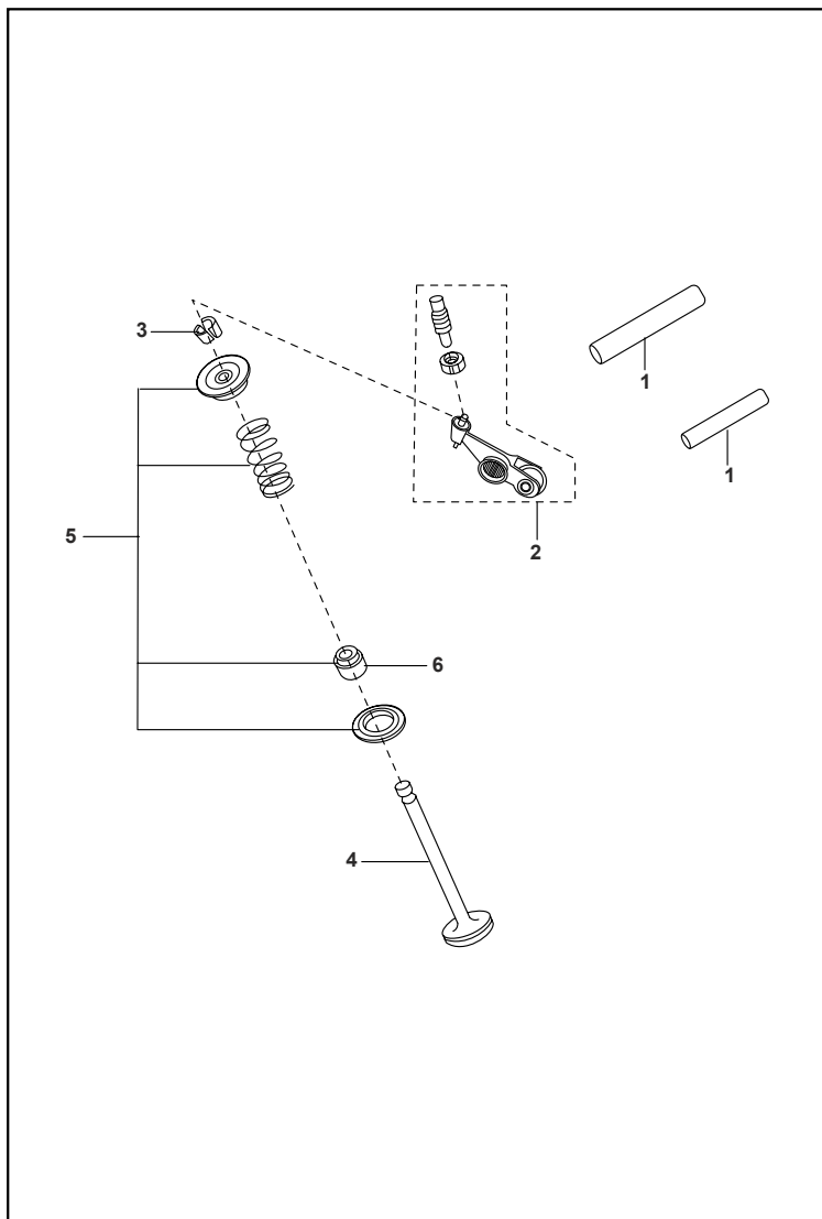
FIGURA Nº 3 : VÁLVULAS
