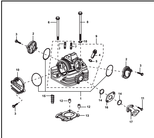
FIGURA N° 1 : CULATA
