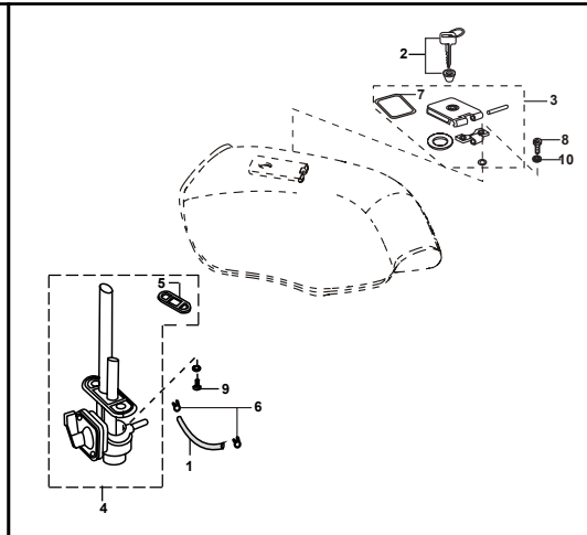
FIGURA N° 32 : TAPA TANQUE DE GASOLINA
