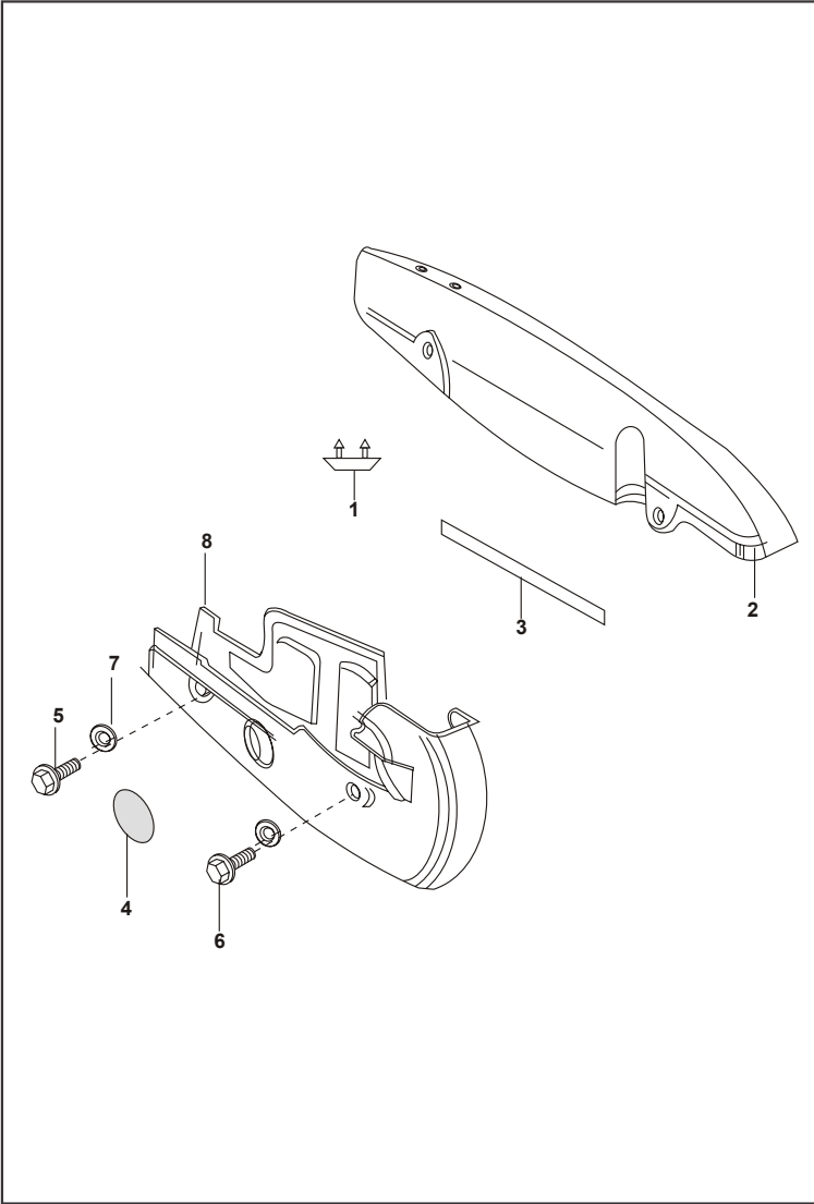
FIGURA N° 33 : CUBIERTA CADENA
