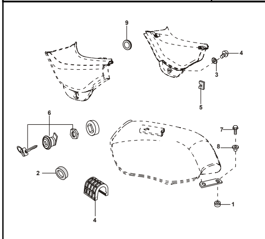
FIGURA N° 34 : ANTIVIBRANTES TANQUE GASOLINA Y TAPAS LATERALES
