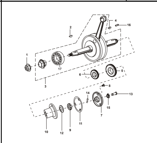
FIGURA N° 5 : CIGÜEÑAL
