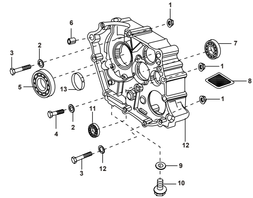
FIGURA Nº 9 : CARCASA DERECHA
