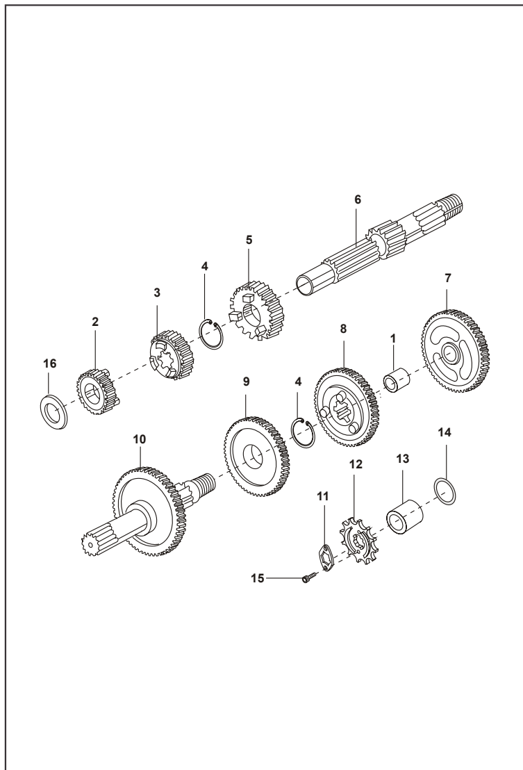
FIGURA N° 6 : TRANSMISIÓN
