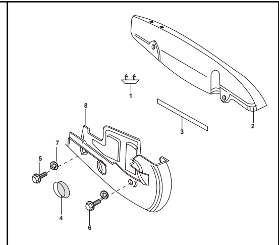
FIGURA N° 33 : CUBIERTA CADENA
