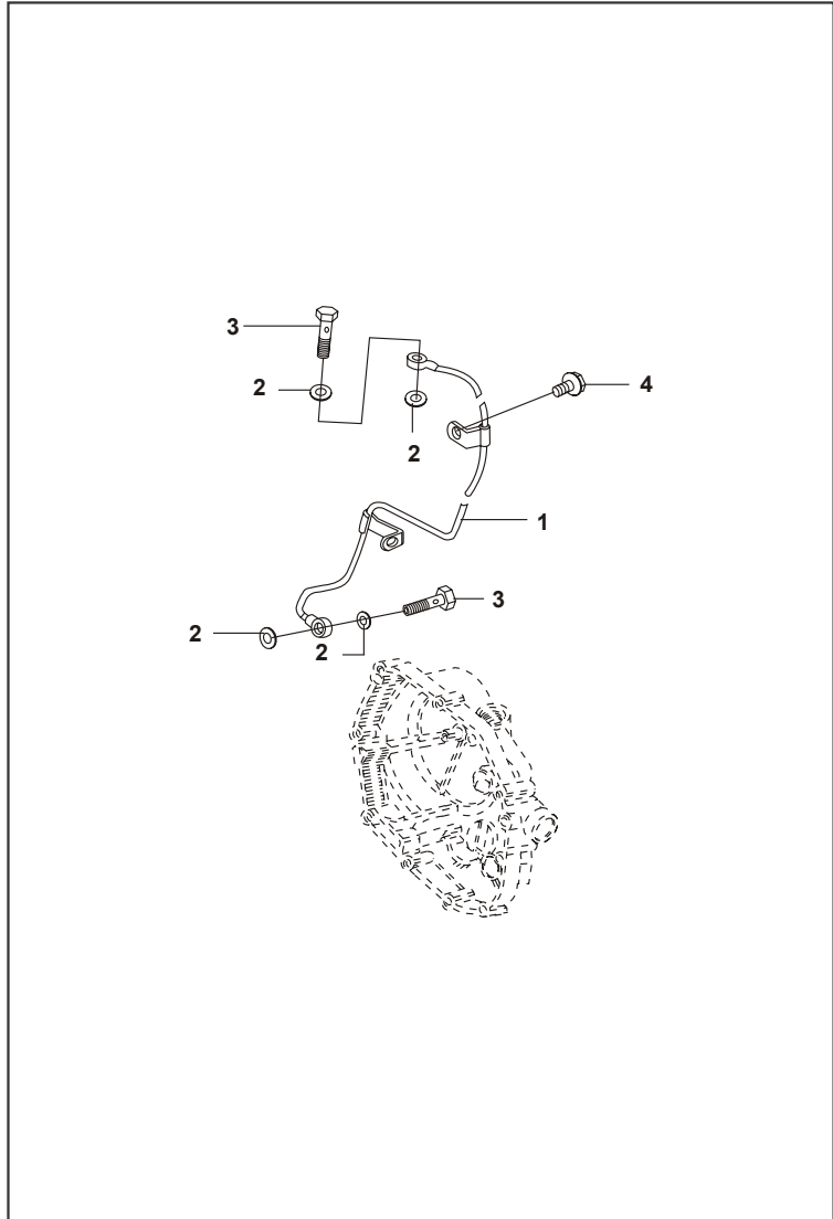
FIGURA N° 11 : CONDUCTO ACEITE
