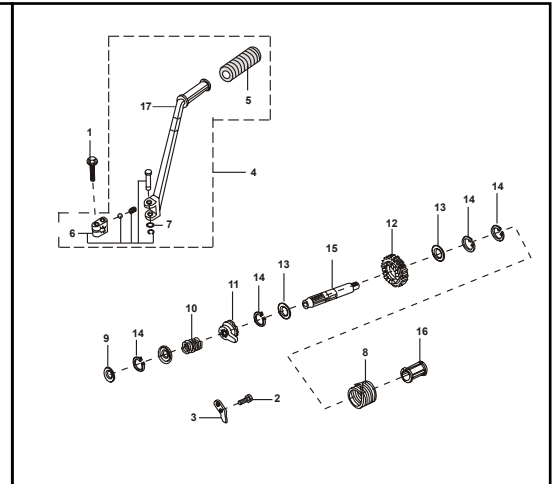
FIGURA N° 15 : PEDAL CRANK
