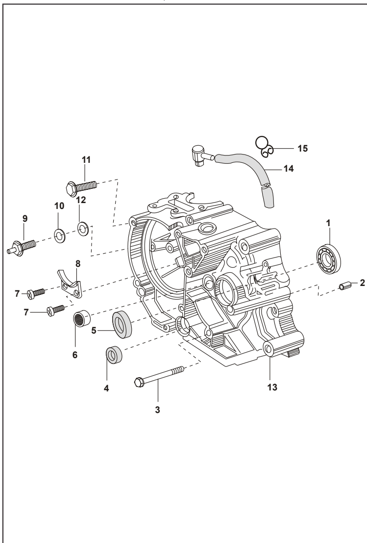
FIGURA N° 10 : CARCASA IZQUIERDA
