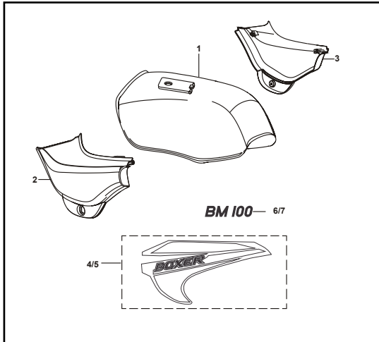
FIGURA N° 31 : TANQUE GASOLINA/ TAPAS LATERALES
