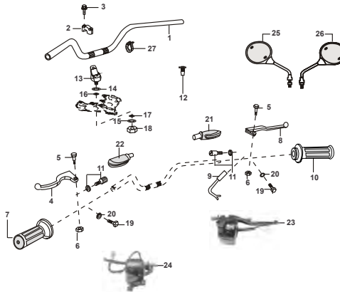
FIGURA N° 29 : MANUBRIO
