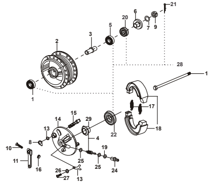
FIGURA N° 26 : CAMPANA DELANTERA
