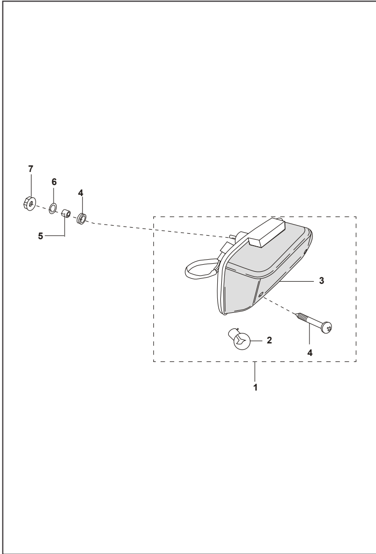
FIGURA N° 40 : STOP
