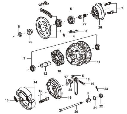
FIGURA N° 27 : CAMPANA TRASERA
