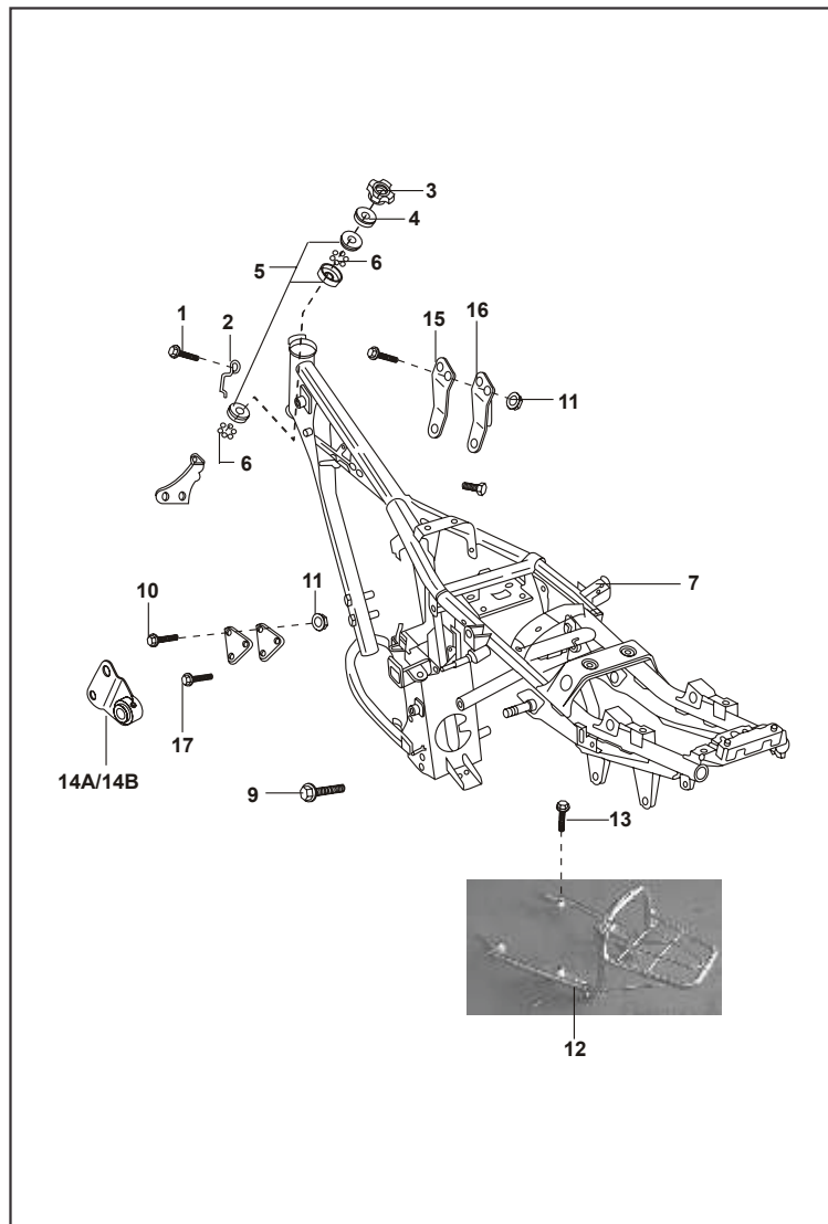
FIGURA N° 21 : CHASIS
