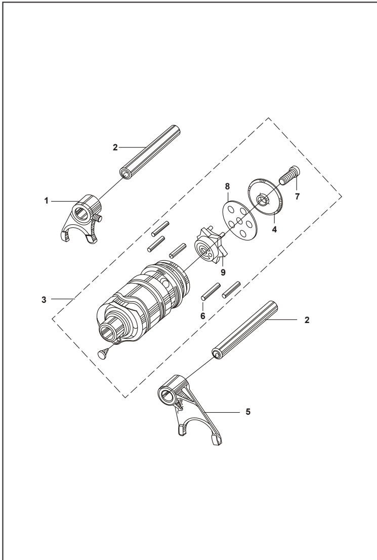
FIGURA N° 7 : SELECTOR CAMBIOS
