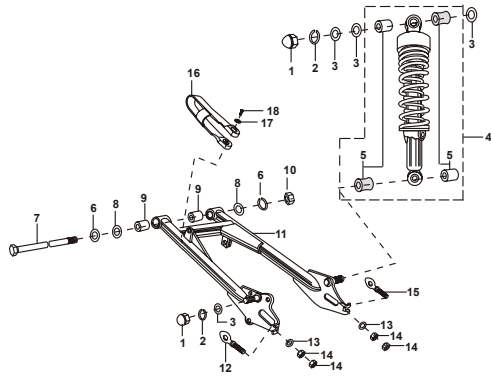
FIGURA Nº 22 : BRAZO OSCILANTE Y AMORTIGUADOR
