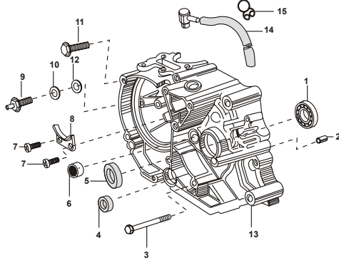
FIGURA Nº 10 : CARCASA IZQUIERDA
