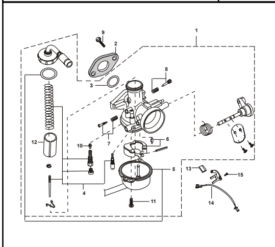
FIGURA N° 16 : CARBURADOR
