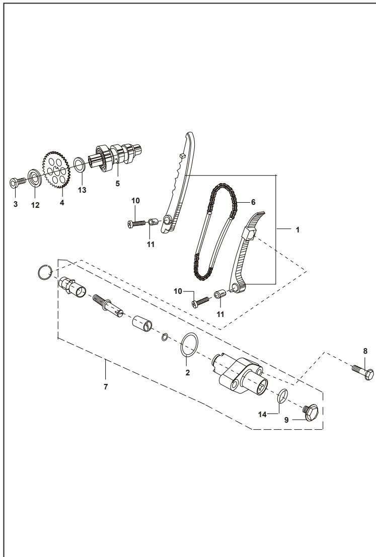
FIGURA N° 3 : EJE DE LEVAS / TENSOR
