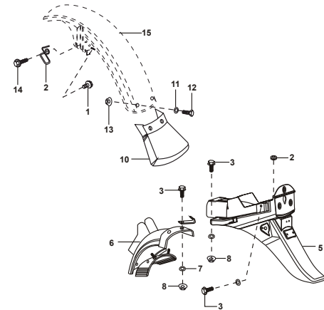
FIGURA Nº 24 : GUARDABARRO DELANTERO Y TRASERO
