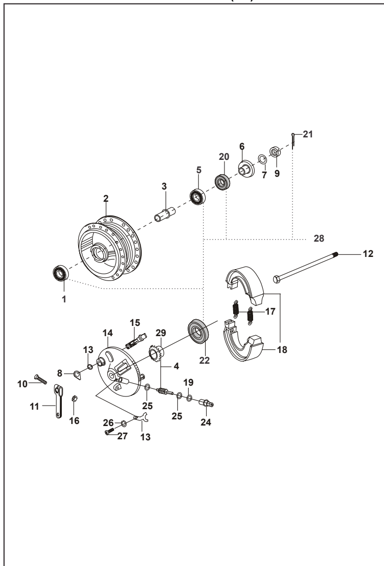
FIGURA N° 26 : CAMPANA DELANTERA (1/2)
