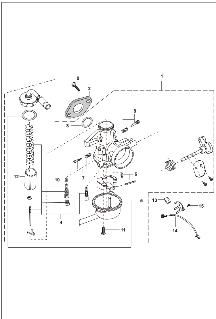
FIGURA N° 16 : CARBURADOR
