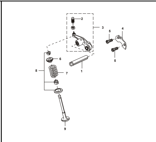
FIGURA N° 2 : VÁLVULAS
