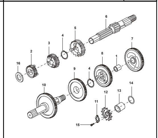
FIGURA N° 6 : TRANSMISIÓN
