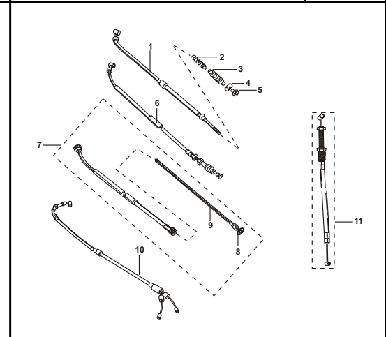
FIGURA N° 36 : CABLES
