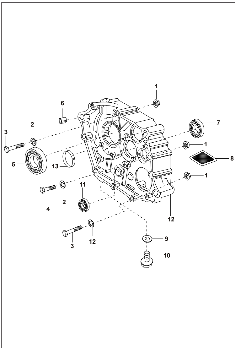
FIGURA N° 9 : CARCASA DERECHA
