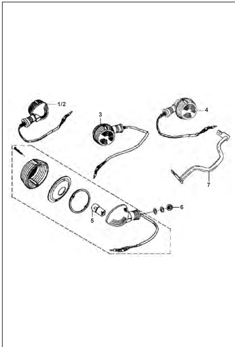
FIGURA N° 38 : DIRECCIONALES
