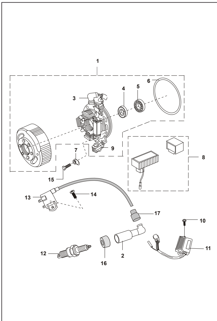
FIGURA N° 20 : PLATO DE BOBINAS
