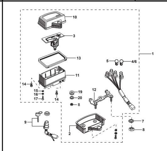
FIGURA N° 35 : VELOCÍMETRO
