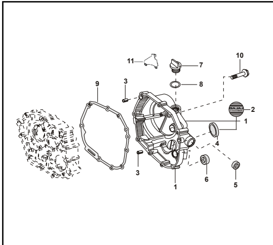
FIGURA N° 13 : CUBIERTA CLUTCH
