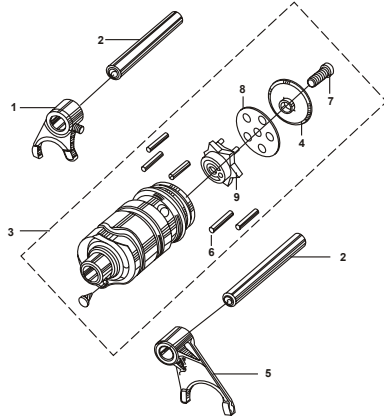
FIGURA Nº 7 : SELECTOR CAMBIOS
