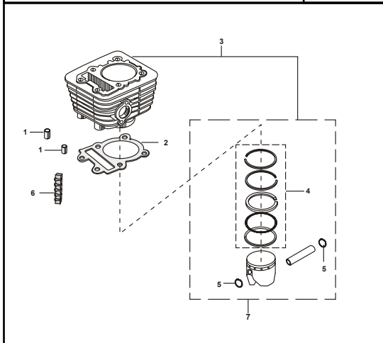
FIGURA N° 4 : CILINDRO Y PISTÓN
