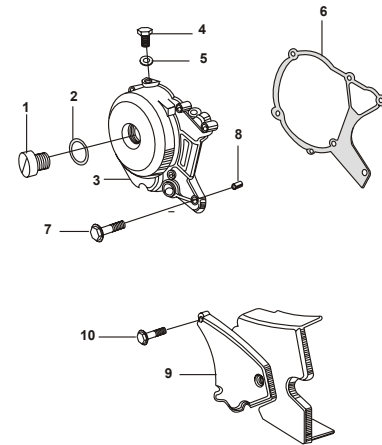
FIGURA Nº 12 : CUBIERTA VOLANTE Y CUBIERTA CADENA
