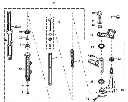
FIGURA N° 30 : SUSPENSIÓN DELANTERA
