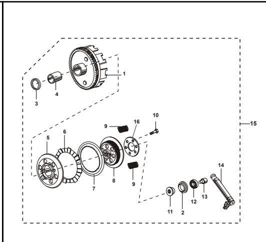
FIGURA N° 14: CLUTCH
