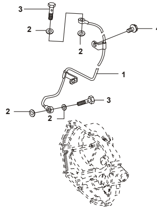
FIGURA Nº 11 : CONDUCTO ACEITE
