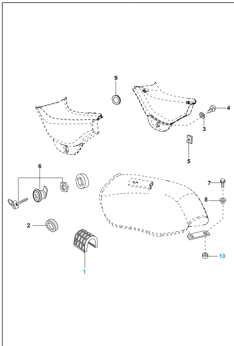
FIGURA N° 34 : ANTIVIBRANTES TANQUE GASOLINA Y TAPAS LATERALES
