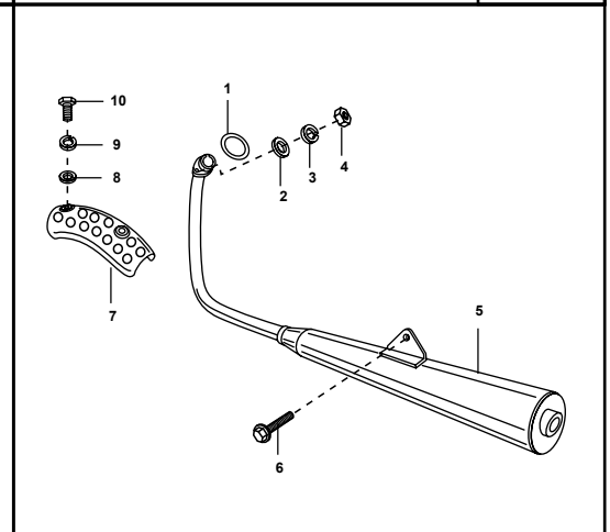
FIGURA N° 18 : SILENCIADOR
