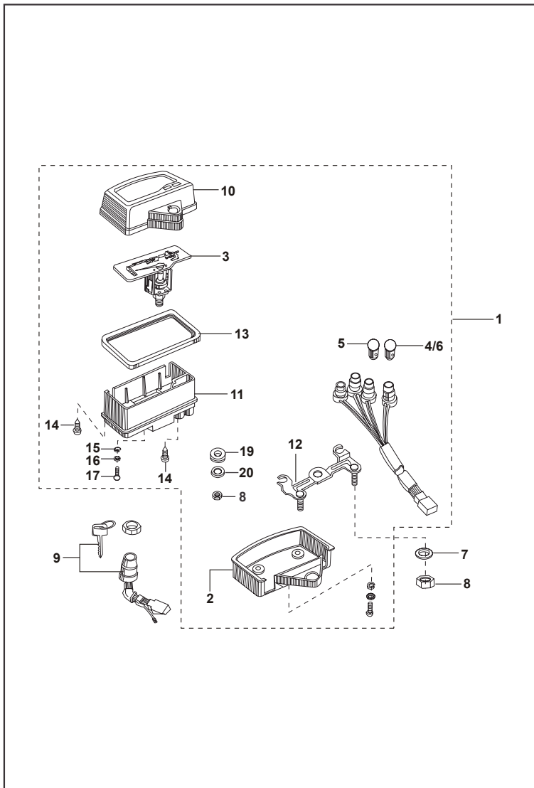
FIGURA N° 35 : VELOCIMETRO
