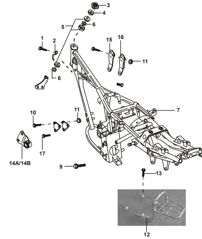
FIGURA Nº 21 : CHASIS
